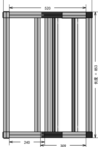
顶视图
